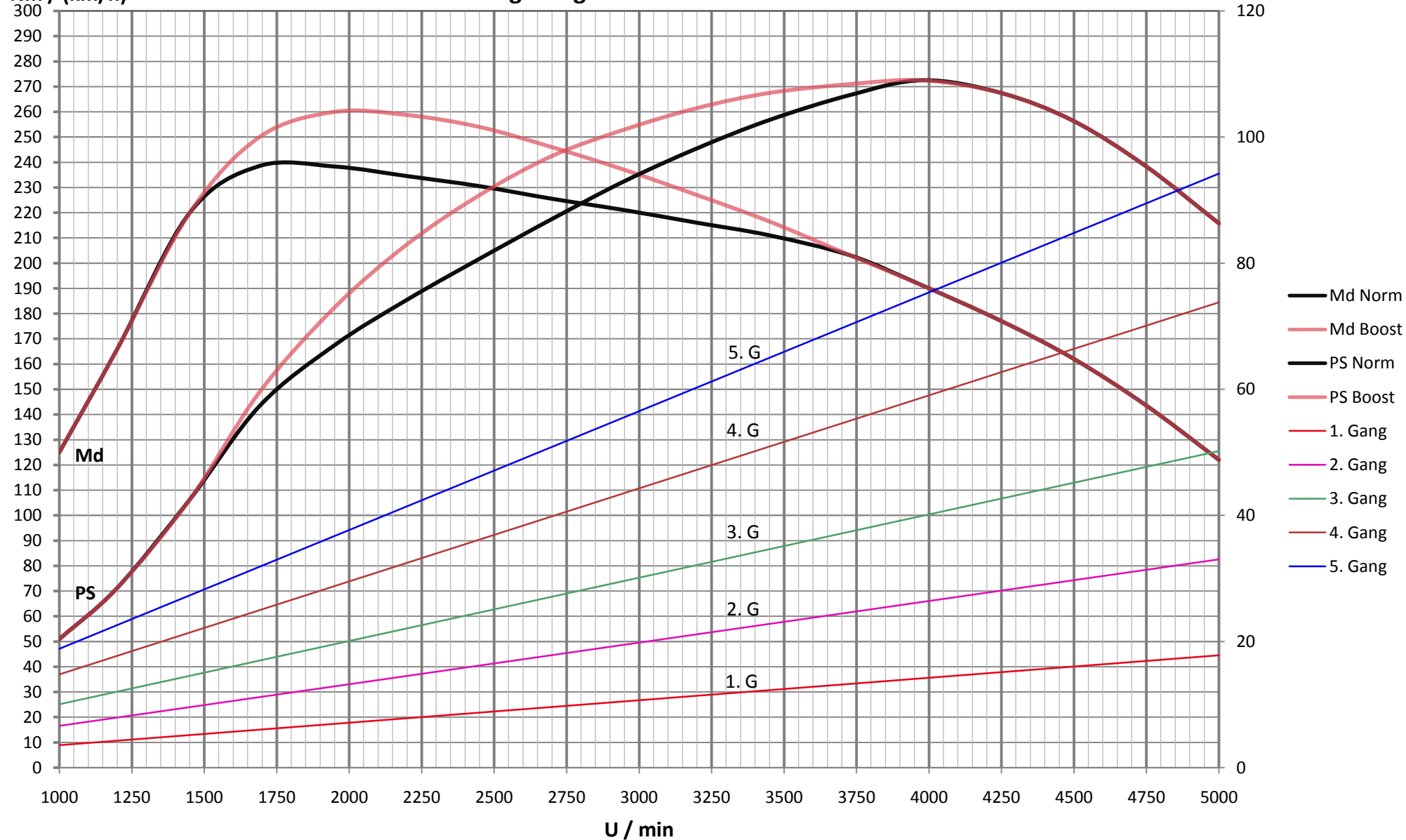
Drehmoment-Leistung-Gangreichweite 1.6 TDCI 109 PS
